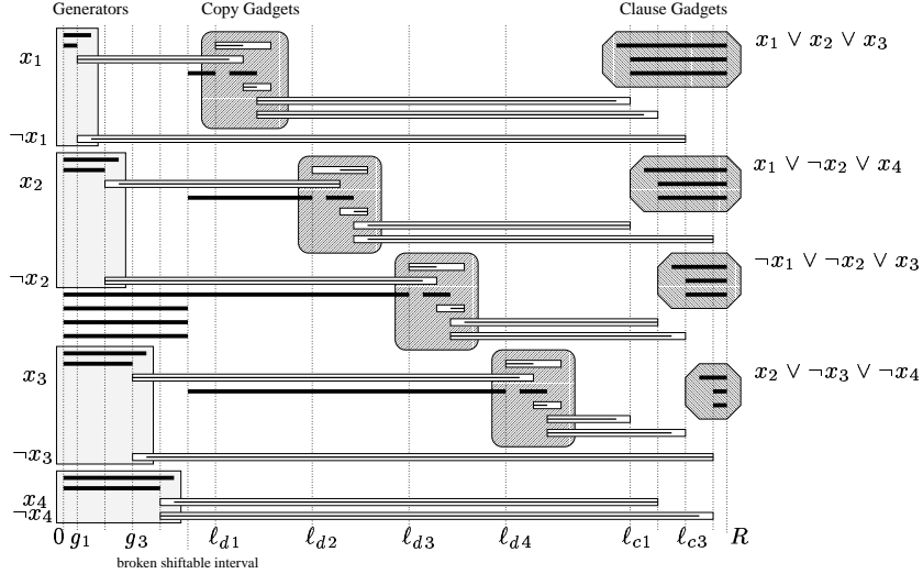
Figure 1. (x_1 \vee x_2 \vee x_3) \wedge (x_1 \vee \neg x_2 \vee x_4) \wedge (\neg x_1 \vee \neg x_2 \vee x_3) \wedge (x_2 \vee \neg x_3 \vee \neg x_4)
