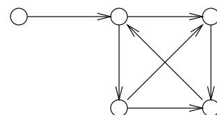
gerichteter Graph
